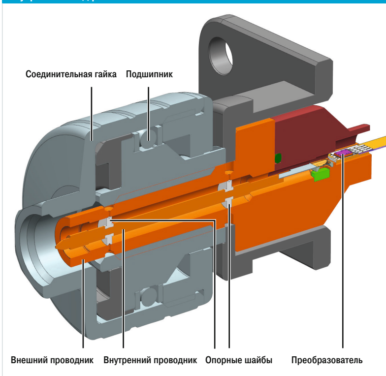
Внутренний вид разъема
