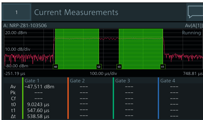
Определение мощности пакетного сигнала EDGE с помощью трехканального диодного датчика мощности R&S®NRPxxS(N) и функции стробирования; исключение тренировочной последовательности в центре сигнала
