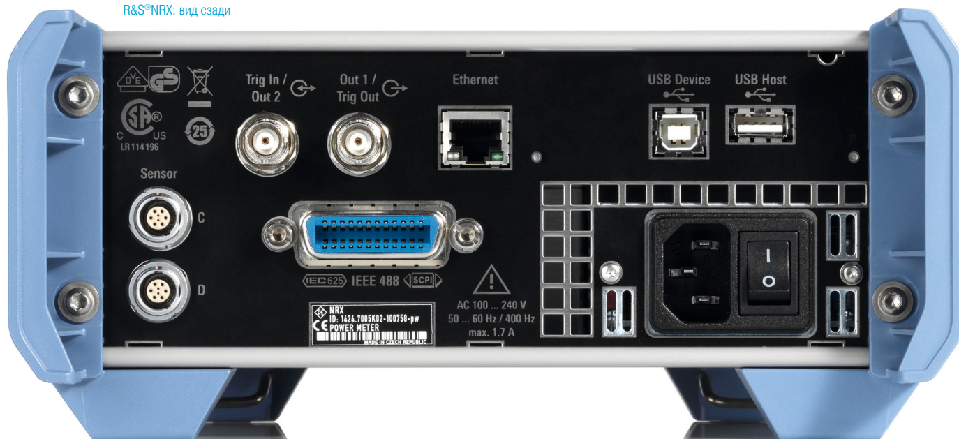
R&S®NRX: вид сзади
