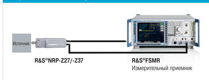
Измерительный приемник R&S®FSMR с модулем датчика мощности R&S®NRP-Z27/-Z37
