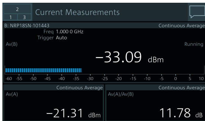
На экране R&S®NRX отображается до четырех измерений одновременно
