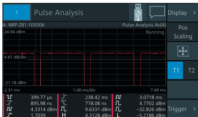
Автоматический анализ импульсов с помощью R&S®NRX и R&S®NRP-Z81
