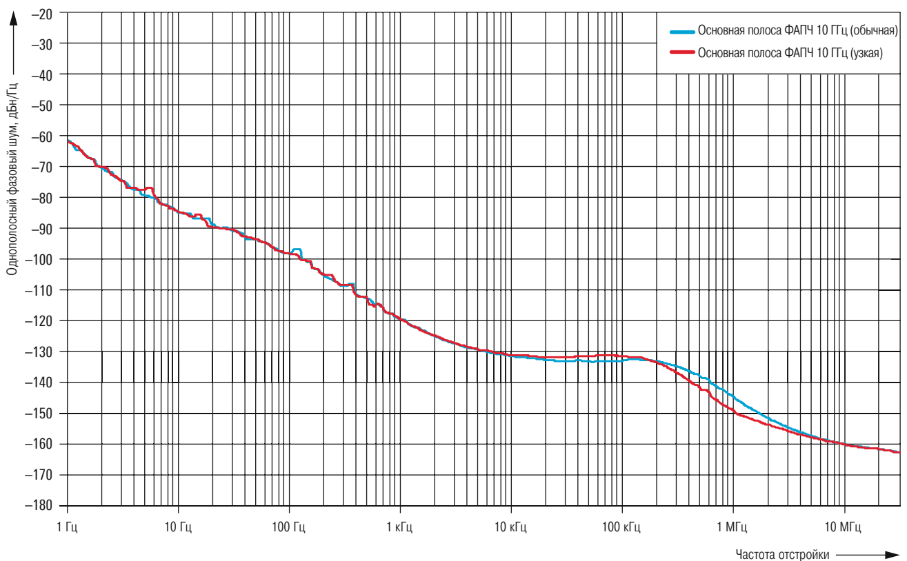
Сравнение характеристик однополосного фазового шума
