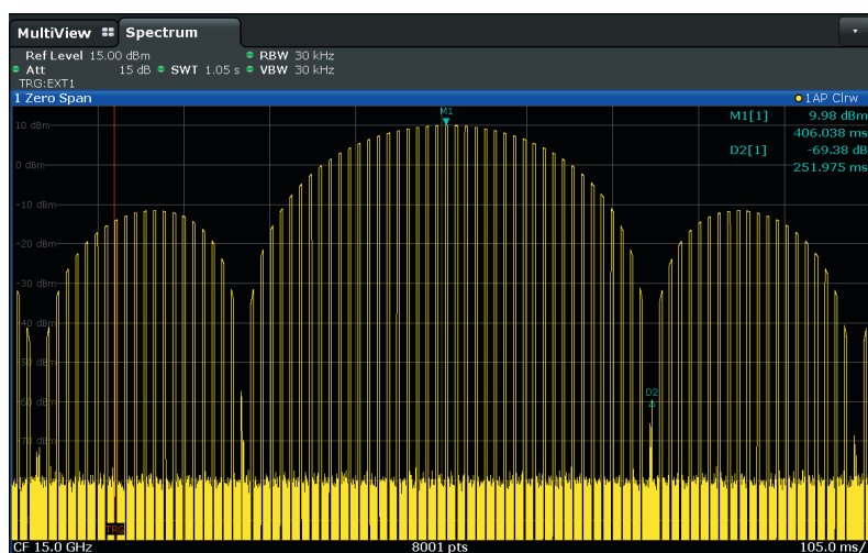
Сигнал с импульсной и амплитудной модуляцией, сформированный генератором R&S®SMA100B. Сигнал модуляции \sin(x)/x подается на вход внешней аналоговой модуляции и формирует сигнал с коэффициентом модуляции 70 дБ (изм.).
