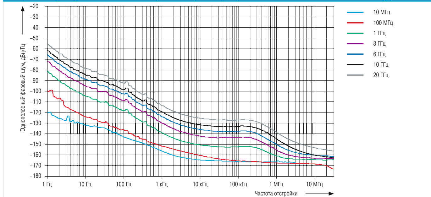
Измеренные характеристики однополосного фазового шума генератора R&S®SMA100B с опцией R&S®SMAB-B711(N)
