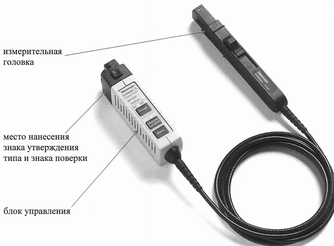
Рисунок 1 – Общий вид пробников токовых ТСП0030А
