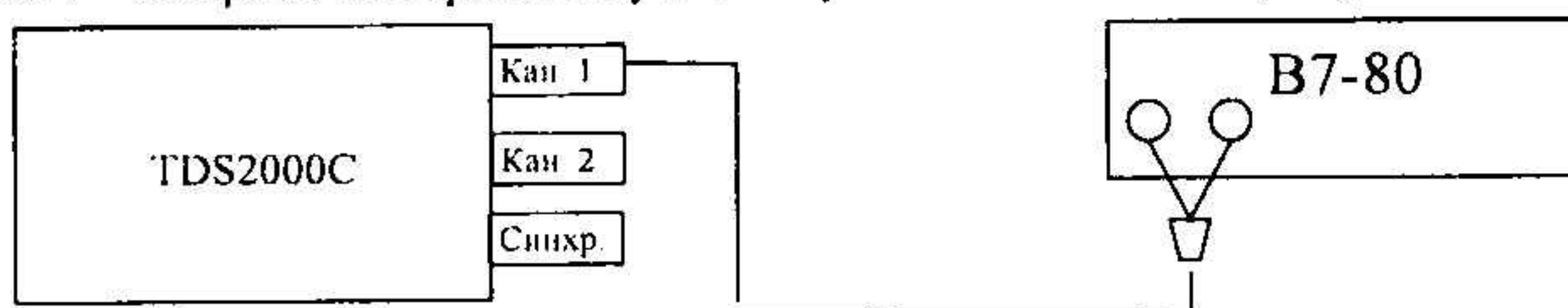
Рисунок 4- Схема определения входного сопротивления
