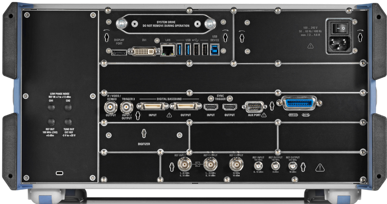
R&S®FSWP: вид сзади
