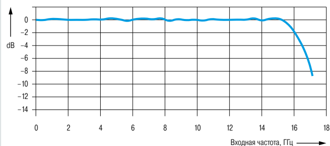
Плоская частотная характеристика осциллографа R&S®RTP164
