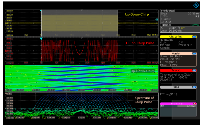
Импульсный анализ ЛЧМ-сигналов во временной и частотной областях с помощью функций осциллографа R&S®RTP
