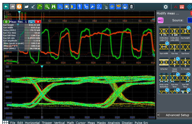
Измерение глазковой диаграммы информационного сигнала памяти DDR
