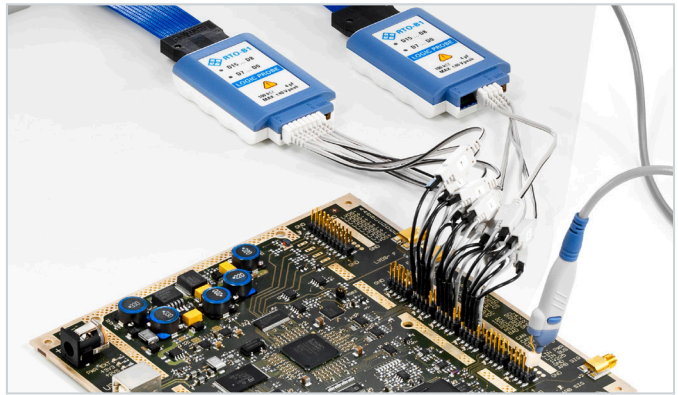
Каждый осциллограф R&S®RTP может быть оснащен дополнительными 16 цифровыми каналами прямо на месте эксплуатации
