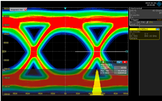
Функции запуска по шаблону высокоскоростных последовательных шин и аппаратного CDR обеспечивают быстрое измерение глазковых диаграмм
