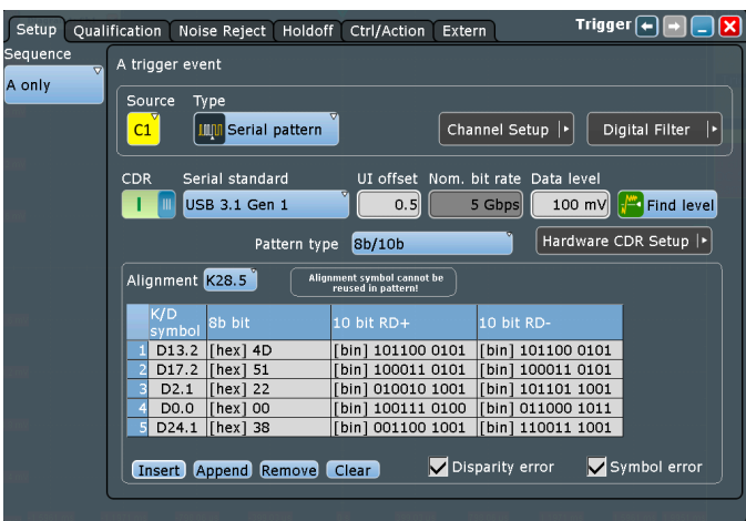
Диалоговое окно настройки запуска по шаблону высокоскоростных последовательных шин
